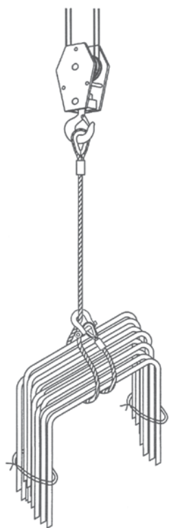
圖 12 單扼雙網索結
