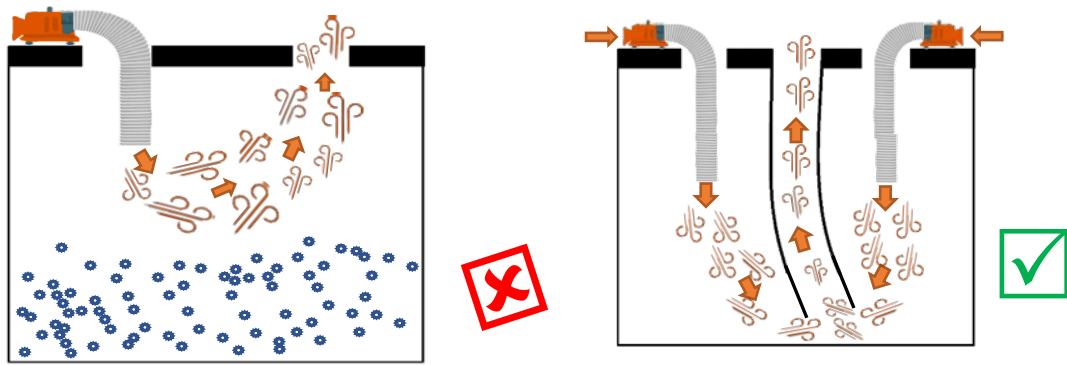
圖 3: 留意通風設備排氣裝置的位置，避免氣流短路。
