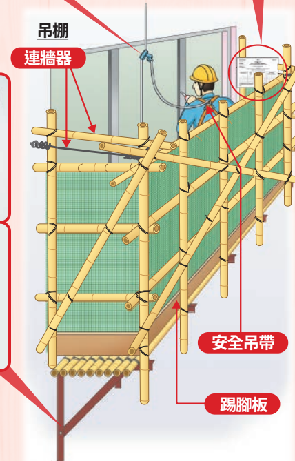
狗臂架必須裝上最少三顆繫穩螺絲
