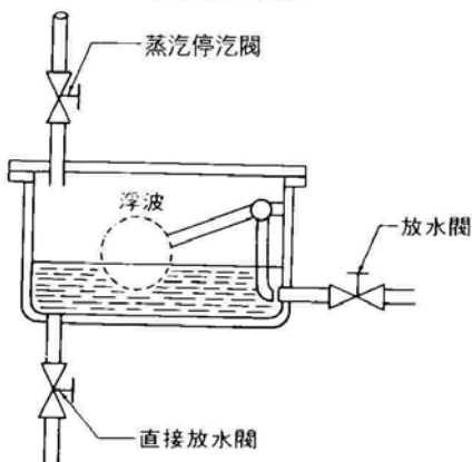
水汽分離器
